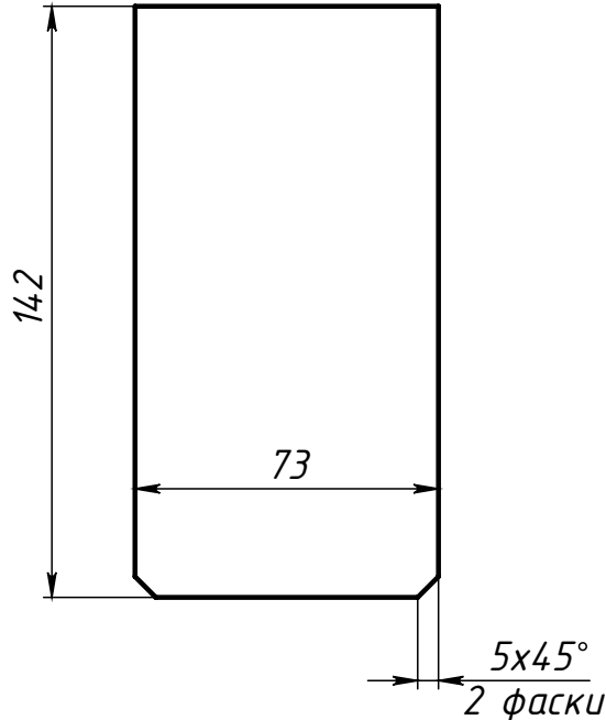
Поз.2 (Ребро)
